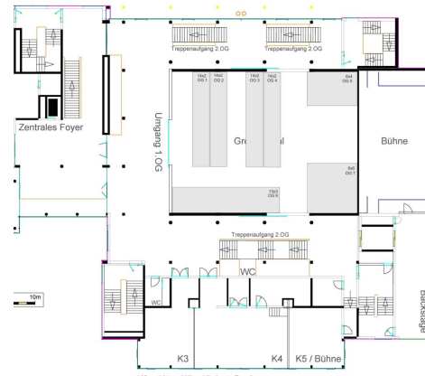
1. Obergeschoss
